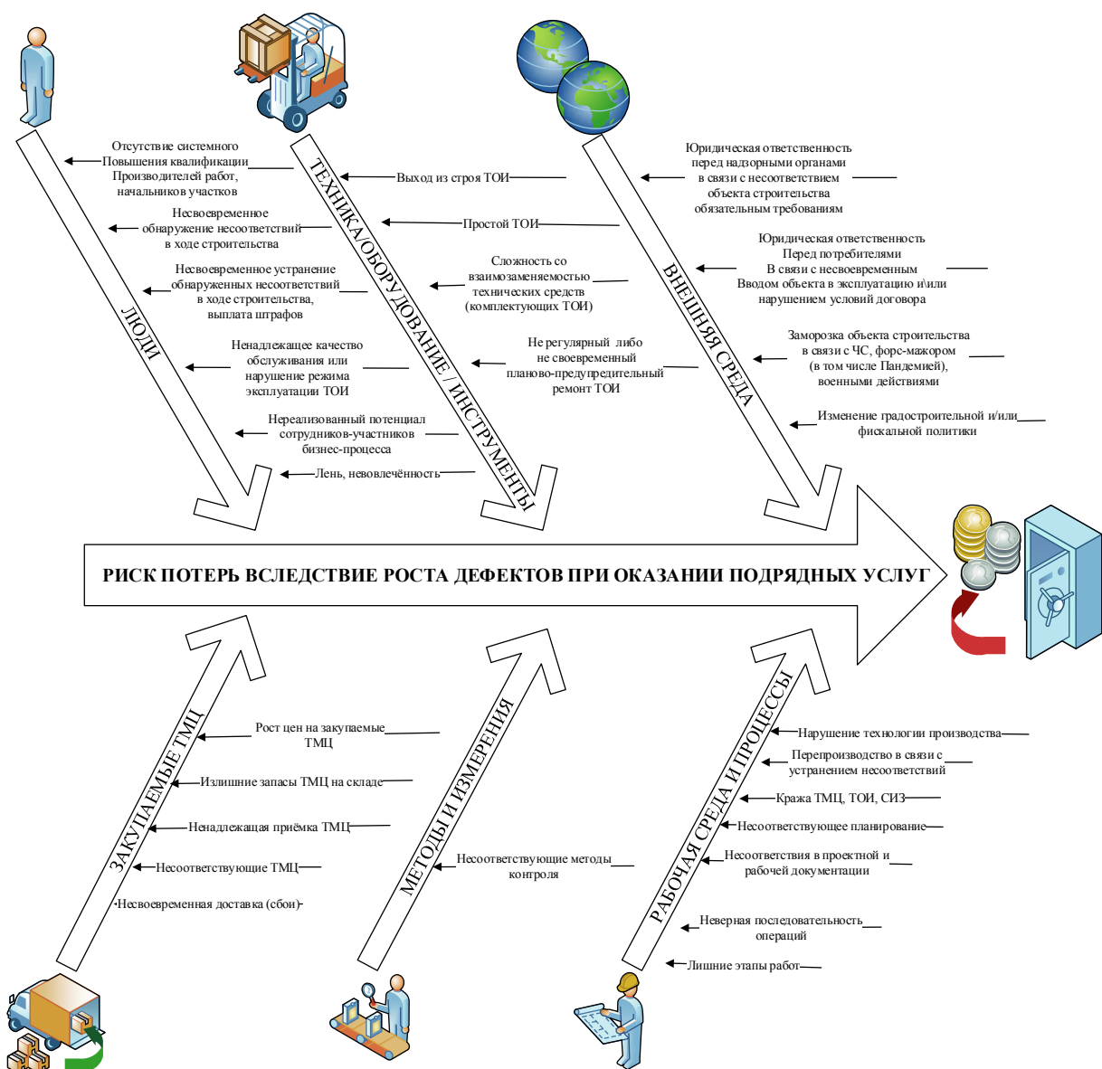
Рисунок 7. Иконографическая модель Диаграммы Исикавы потенциальных областей потерь и причин повышения себестоимости многоэтажного домостроения при менеджменте качества подрядных строительных услуг
