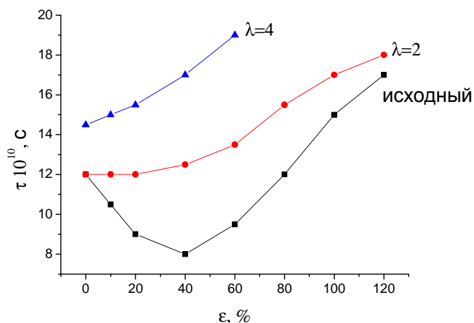
Рис. 4. Зависимости времени корреляции вращения зонда ( \tau ) от степени деформации ( \epsilon ) для ПУ с 0,63 % ХГ, подвергнутых предварительной вытяжке ( \lambda )
