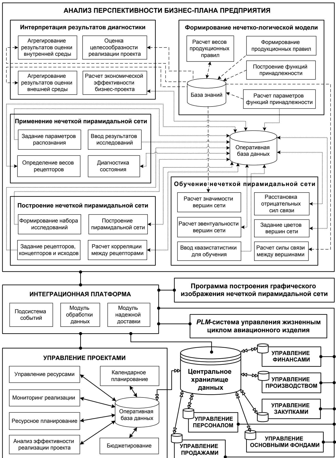
Рисунок 4 – Архитектура экспертно-диагностической системы анализа бизнес-планов авиационного предприятия
