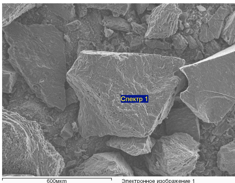
Рис. 4.1. Электронное изображение поверхности карбонизата СКО
