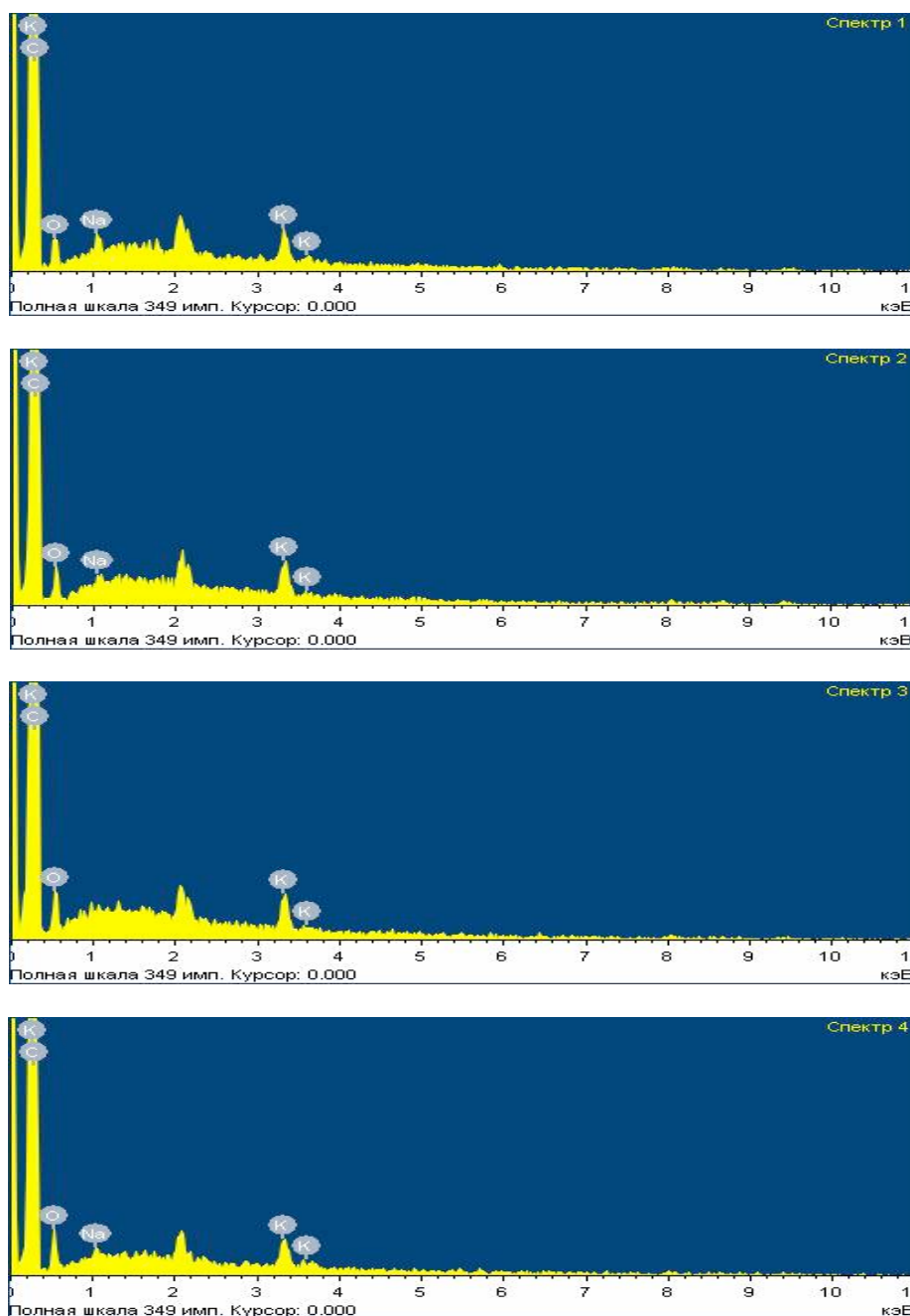
Рис. 4.4. Спектры поверхностных точек активного угля, полученного из СКО (согласно электронного изображения рис. 4.3)
