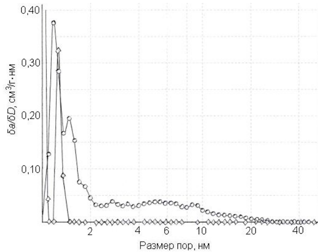
Рис. 4.7. Распределение пор АУ по размерам
