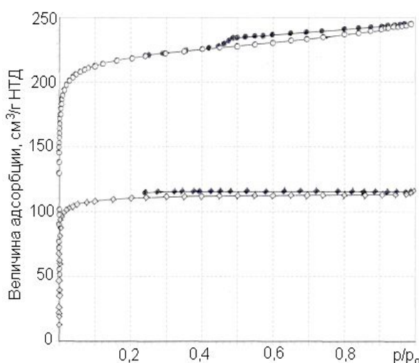
Рис. 4.5. Равновесие адсорбции азота при 77 К: (◇) – КСКО адсорбция, (◆) – КСКО десорбция; (○) – АУ адсорбция, (●) – АУ десорбция
