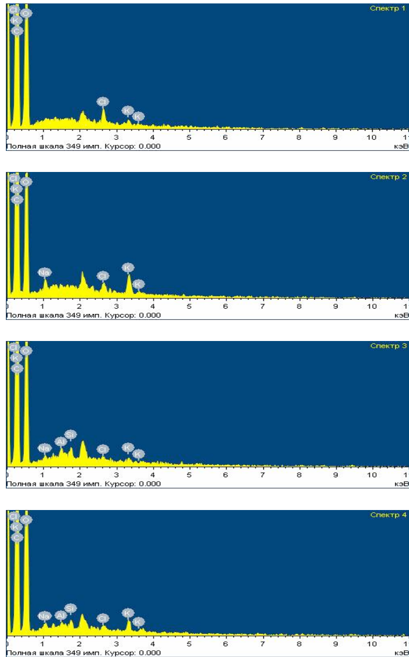
Рис. 2.2. Спектры поверхностных точек фрагмента СКО согласно электронного изображения рис. 2.1.
