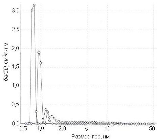
Рис. 4.6. Распределение пор КСКО по размерам
