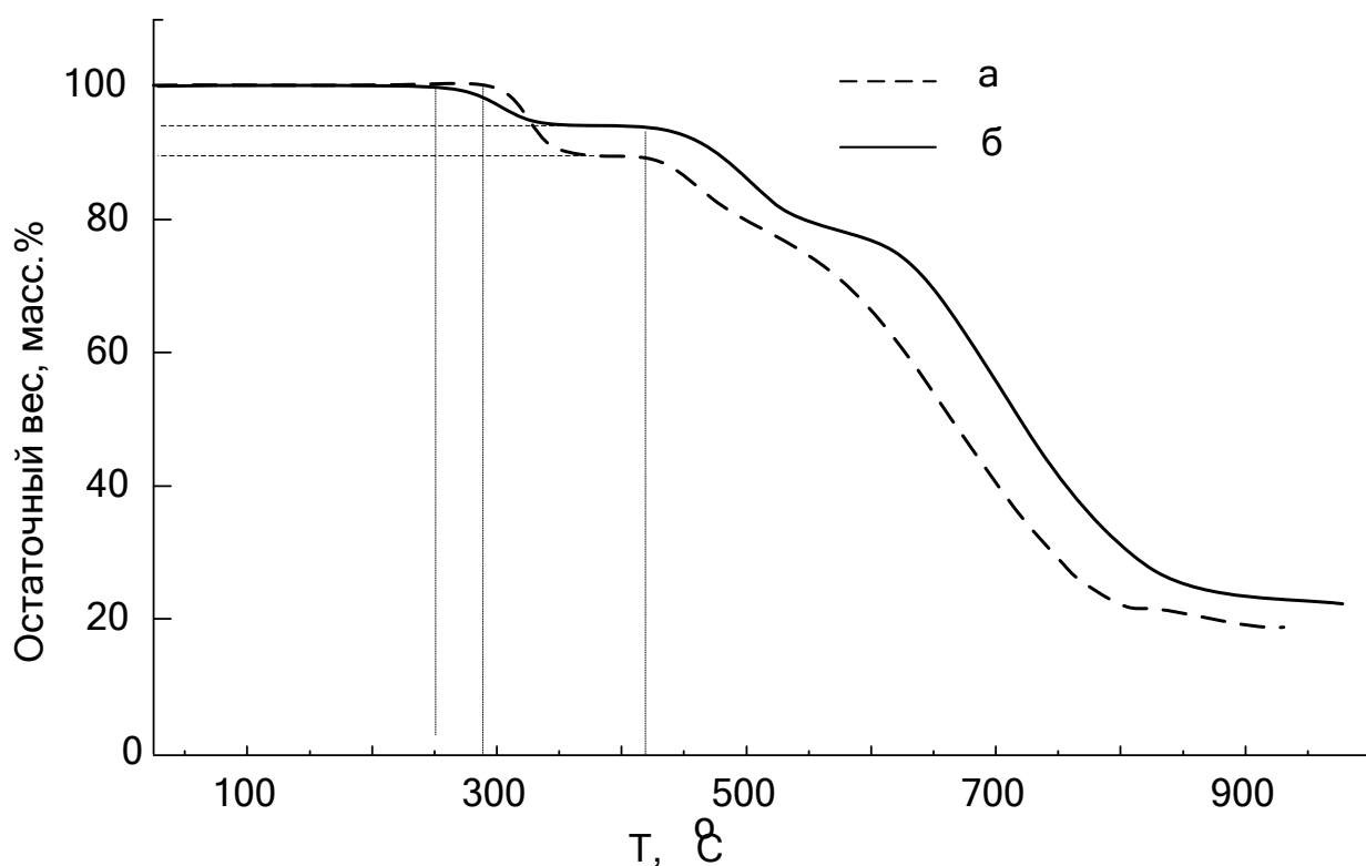
Рисунок 9 - ТГА гривые соединения VII (а) и с добавлением 0.5 масс. % пара-толуолсульфо кислоты (б).
