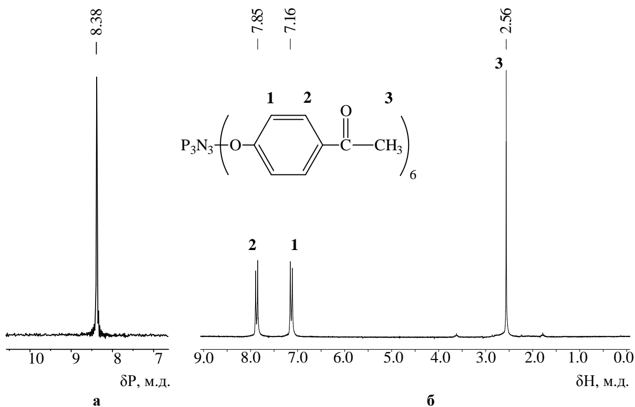
Рисунок 7— ^{31}\text{P} (а) и ^1\text{H} (б) ЯМР-спектры гекса-пара-ацетофеноксциклотрифосфазена.
