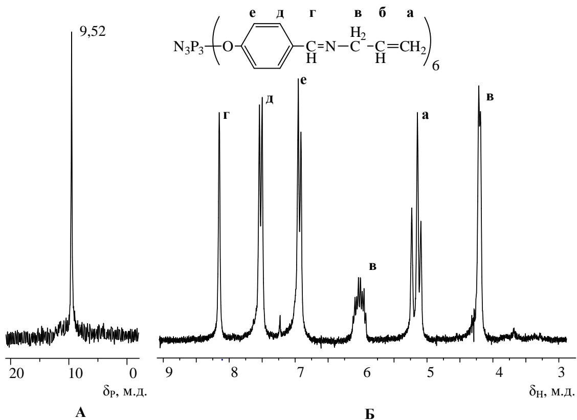
Рисунок 25 – 31 P (А) и 1 H (Б) ЯМР спектры соединения XVII.
