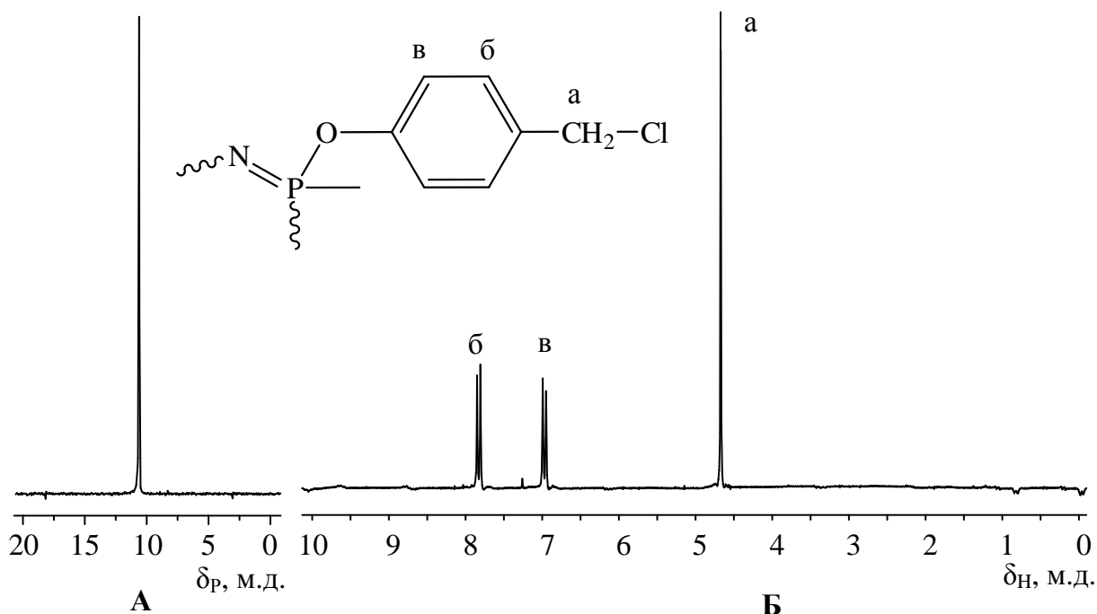
Рисунок 30— 31 P (А) и 1 H (Б) ЯМР спектры соединения XIX.
